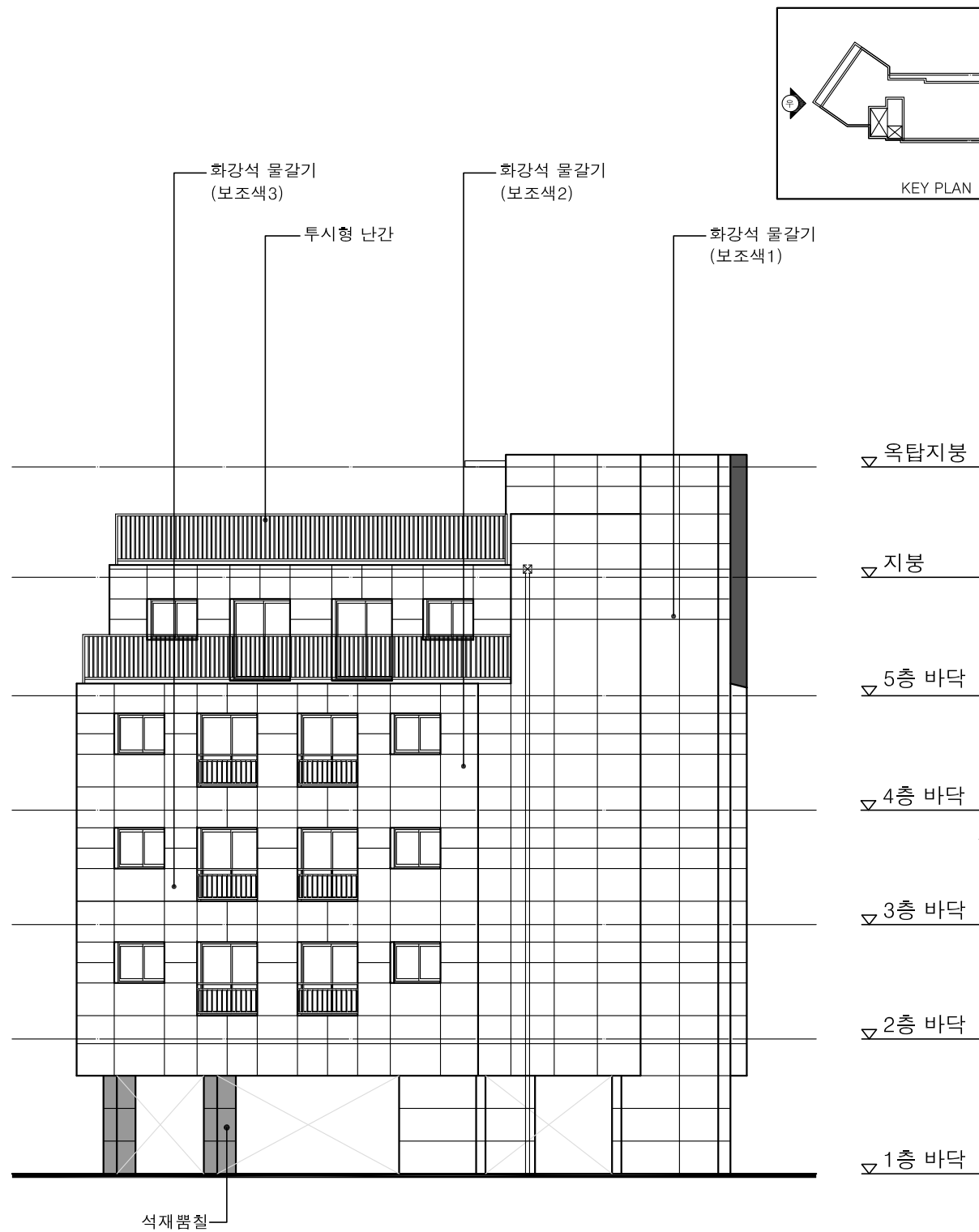
1 우 측 면 도 축척 : 1 / 150
