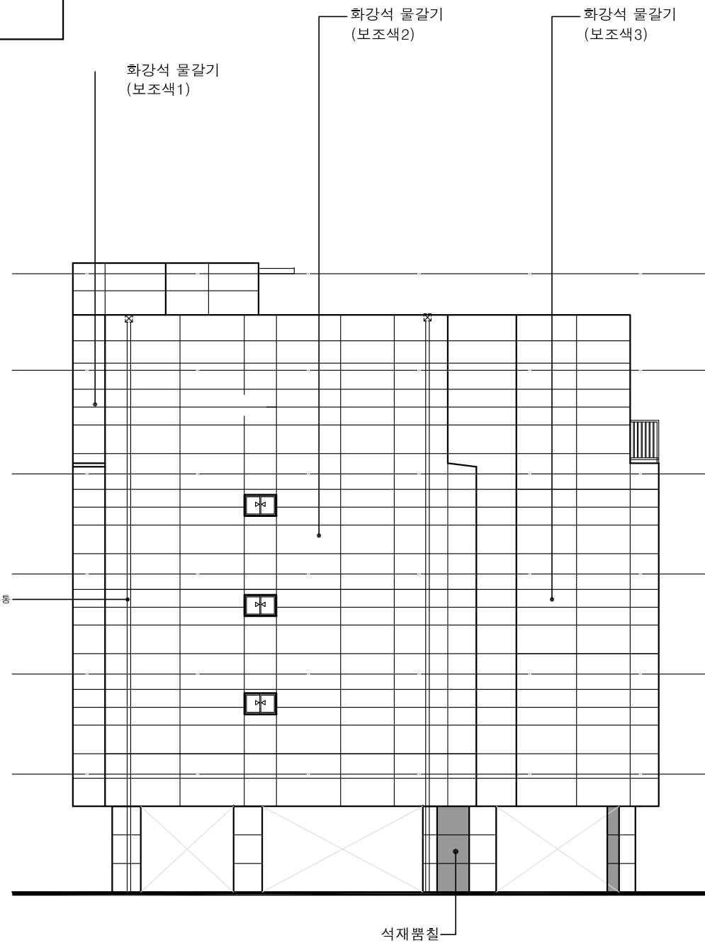
2 좌 측 면 도 축척 : 1 / 150
